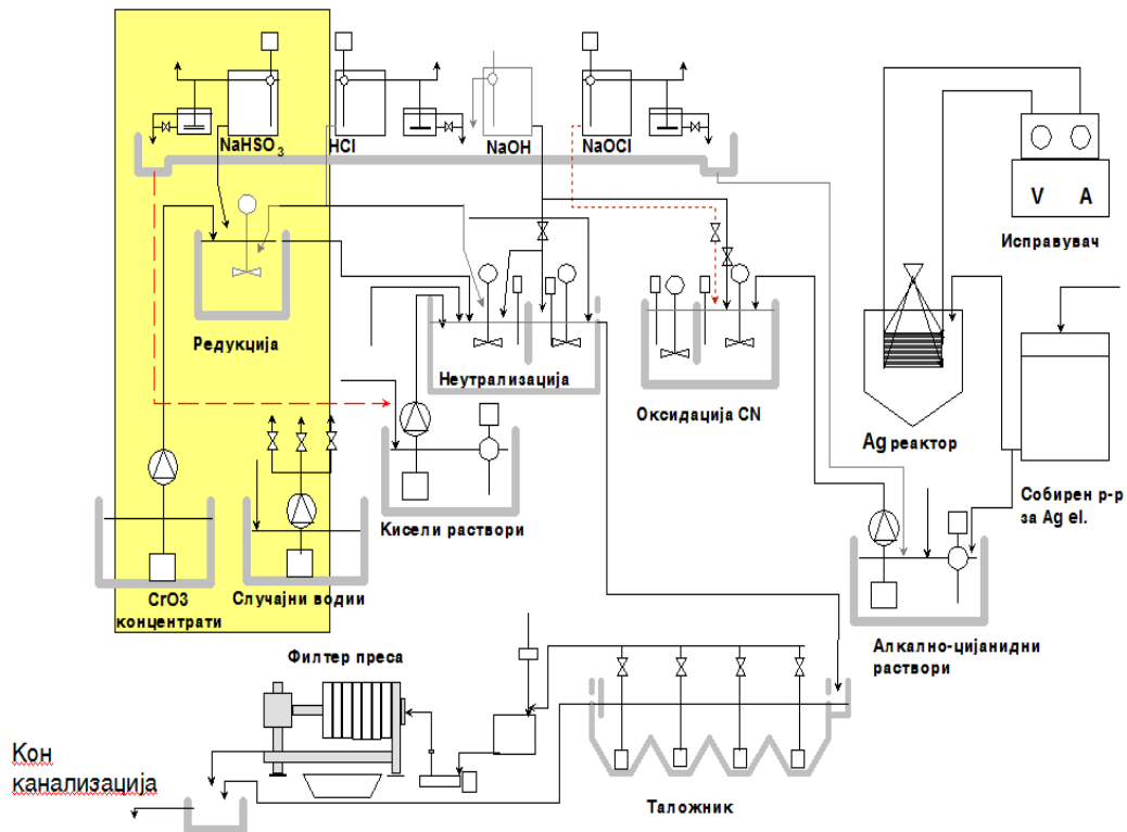
Слика 2. 1 Шема на третманот на отпадните води (пожолтеното поле нема да се користи поради исфрлањето на употребата на Cr 6+ )
